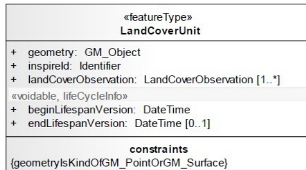
Fig. 4. La clase LandCoverUnit
