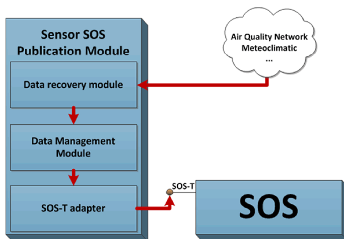
Figura 5: Sensor Módulo de publicación SOS.
