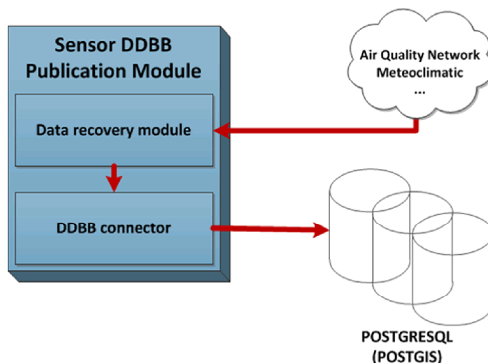
Figura 4: Sensor Módulo de publicación BBDD.
